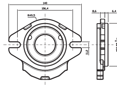
Type flange SAEA-AC Flangia tipo SAEA-AC
