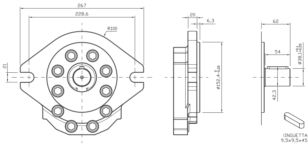
TYPE / TIPO SAED-AC
