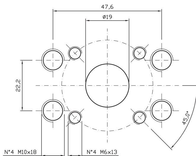
Inlet/Outlet
