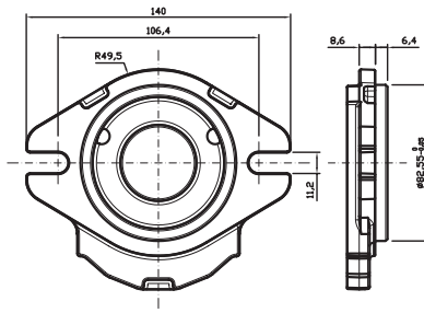
Type flange SAEA-AT11 Flangia tipo SAEA-AT11
