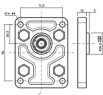
Type flange 2C4 Flangia tipo 2C4
