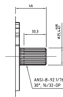
Type shaft SAEB-T15 Albero tipo SAEB-T15 Max torque / Coppia max: 700 Nm
