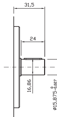
Type shaft SAEA-AC Albero tipo SAEA-AC Max torque/Coppia max: 140 Nm
