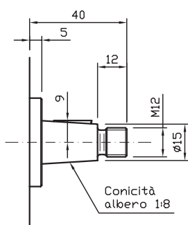
Type shaft 2C4 Albero tipo 2C4
