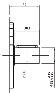
Type shaft SAEB-AC Albero tipo SAEB-AC Max torque / Coppia max: 550 Nm
