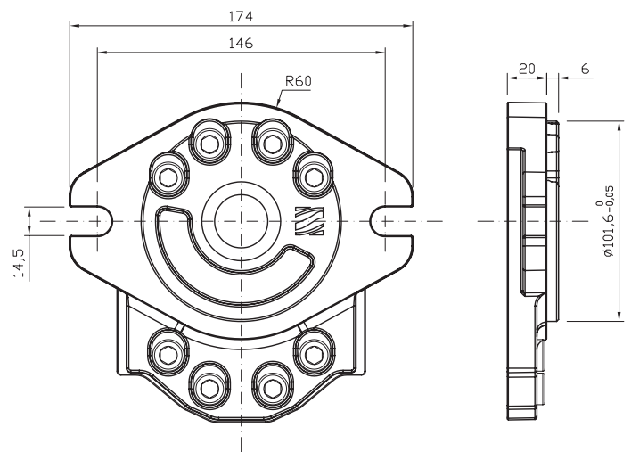
Type flange SAEB-T15 Flangia tipo SAEB-T15
