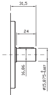
Type shaft SAEA-AC Albero tipo SAEA-AC
