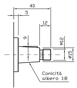
Type shaft 2C4 Albero tipo 2C4 Max torque/Coppia max: 210 Nm
