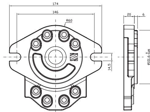
Type flange SAEB-AC Flangia tipo SAEB-AC
