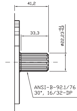
Type shaft SAEB-T13 Albero tipo SAEB-T13 Max torque / Coppia max: 600 Nm
