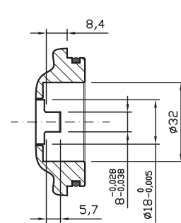
Type shaft 2BK7-G Albero tipo 2BK7-G
