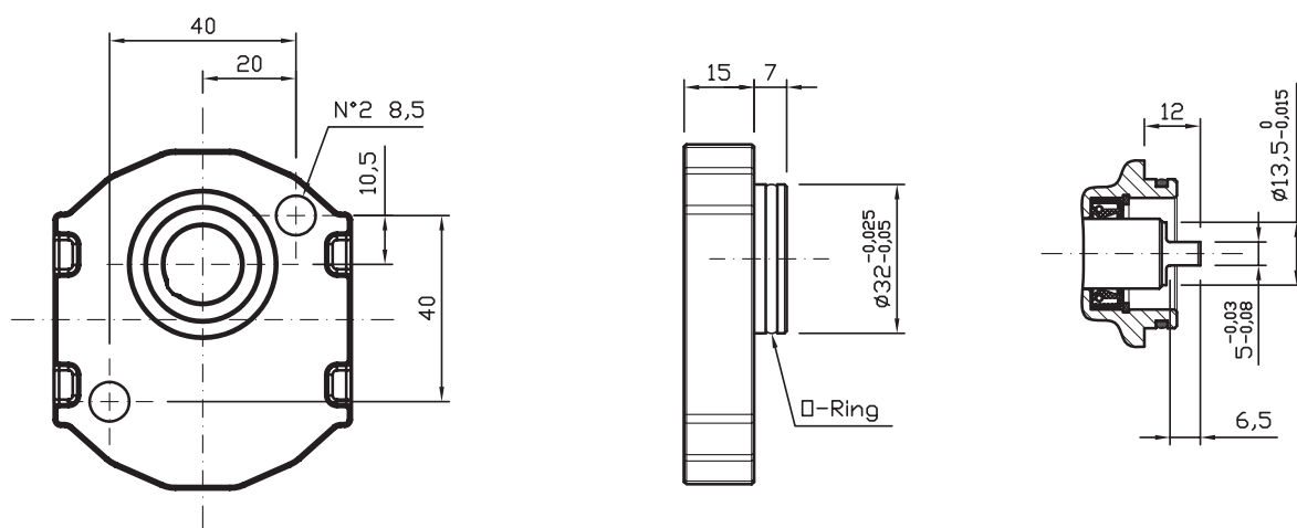
TYPE / TIPO 1K-GL54
