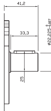
Type shaft SAEB-AC Albero tipo SAEB-AC Max torque / Coppia max: 450 Nm
