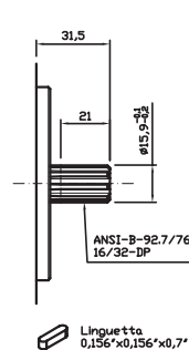
Type shaft SAEA-T9 Albero tipo SAEA-T9
