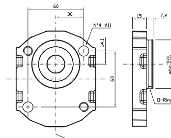
Type flange 2BK7-G Flangia tipo 2BK7-G
