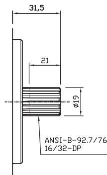
Type shaft SAEA-AT11 Albero tipo SAEA-AT11 Max torque/Coppia max: 210 Nm
