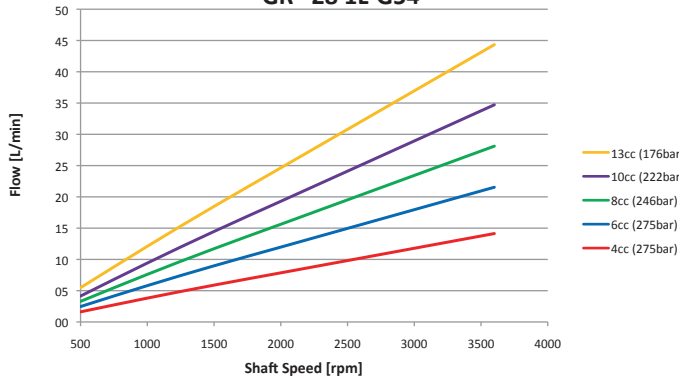
GR 28 1K-G54 GR 28 1K-GL54
