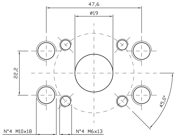
Inlet/Outlet
