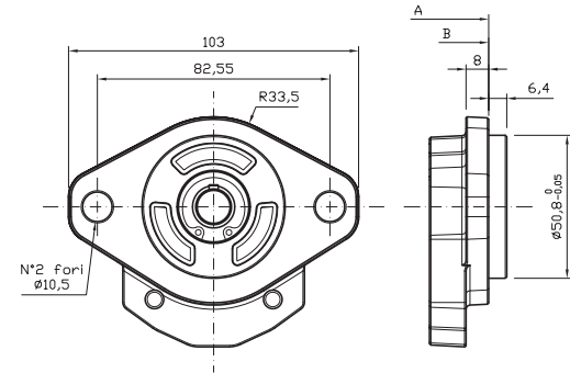
Type flange SAEA-AC Flangia tipo SAEA-AC
